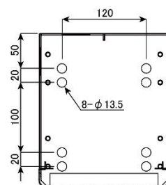
架台アンカー設置 寸法図 (上面視図)
